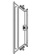
ワイドアングル リプレースメントシェード K5.65585.0 LMB4をLMB-4Aに アップグレード (LMB-4Aは標準装備)
